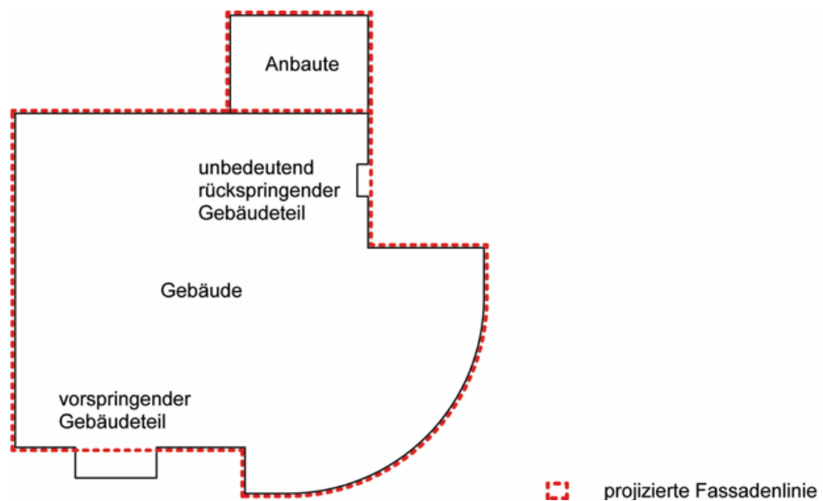
Abbildung 1: Projizierte Fassadenlinie
