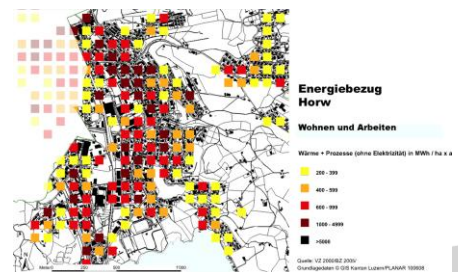
Abb.1: Energiebezug Dienstleistung, Gewerbe und Industrie im ha-Raster (Quelle VZ 2000, BZ 2005), Energieplanung Horw, PLANAR 2011
